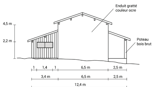
FAÇADE OUEST
